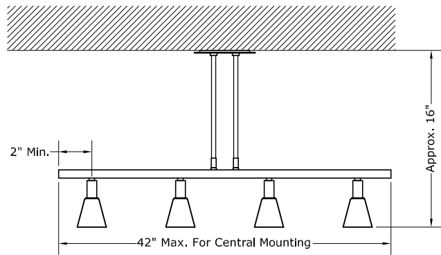
Front View 10" Stem (Specify Stem: 2", 6", 10", 16", or Custom Stem)
