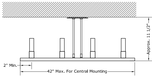
Front View 10" Stem (Specify Stem: 2", 6", 10", 16", or Custom Stem)
